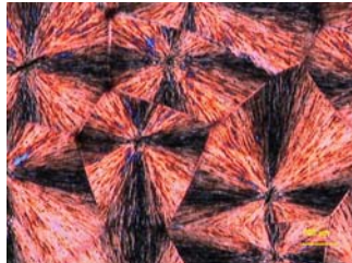
Κρυστάλλωση Πολυμερών
