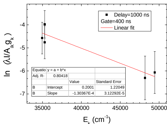
Διάγραμμα 12. Διάγραμμα Boltzmann σε \tau_d = 1000 ns
