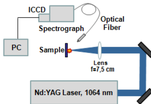
Εικόνα 2. Σχηματικό διάγραμμα της πειραματικής διάταξης που χρησιμοποιήθηκε για την λήψη των φασμάτων LIBS.
