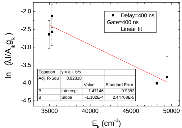
Διάγραμμα 11. Διάγραμμα Boltzmann σε \tau_d = 400 ns
