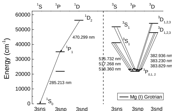
Διάγραμμα 6. Ενεργειακό διάγραμμα Grotrian του Mg I
