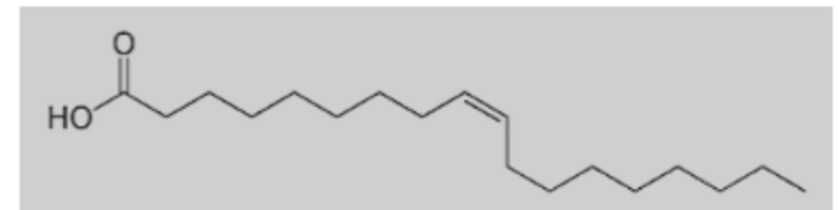
Ελαϊκό οξύ
