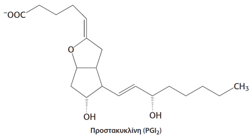
Προστακυκλίνη (PGI 2 )
