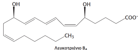
Λευκοτριένιο B 4
