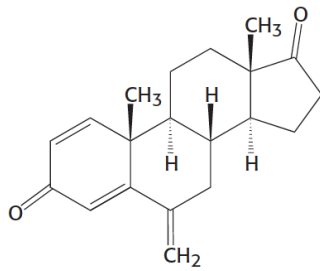
Εξεμεστάνη
