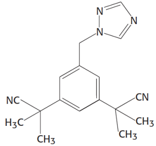
Αναστοζόλη
