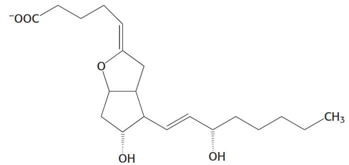
Προστακυκλίνη (PGI 2 )
