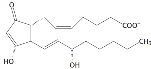
Προσταγλανδίνη E 2
