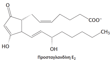
Προσταγλανδίνη E 2
