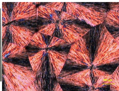
Κρυστάλλωση Πολυμερών
