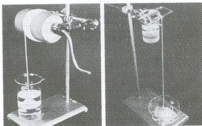
Σύνθεση πολυαμιδίου
